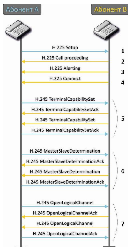
Рисунок 14 – Алгоритм вызова по протоколу H.323
