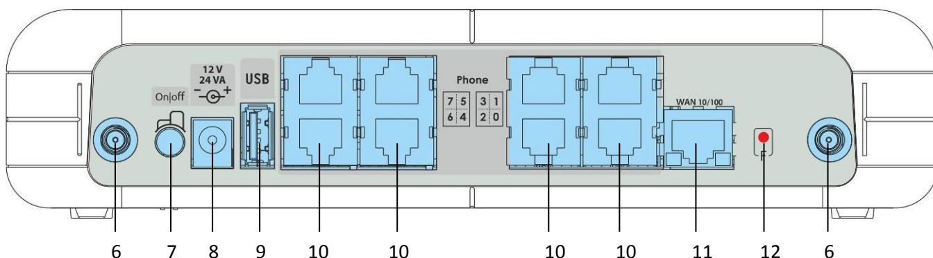
Рисунок 5 – Внешний вид задней панели TAU-8.IP-W
