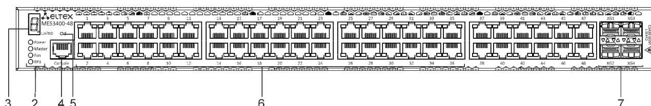
Рисунок 28 – Передняя панель MES3400-48
