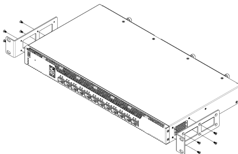
Рисунок 56 – Вариант крепления кронштейнов №1
