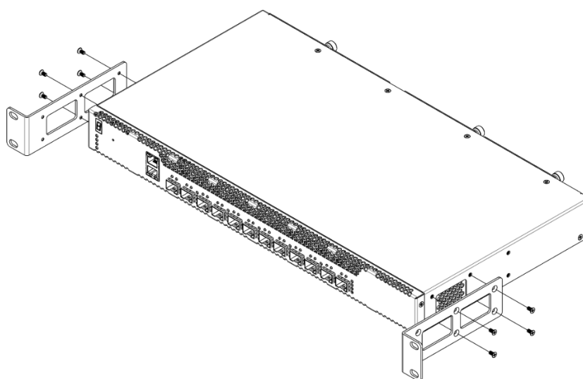
Рисунок 57 – Вариант крепления кронштейнов №2
