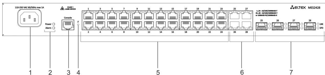
Рисунок 12 – Передняя панель MES2428 AC
