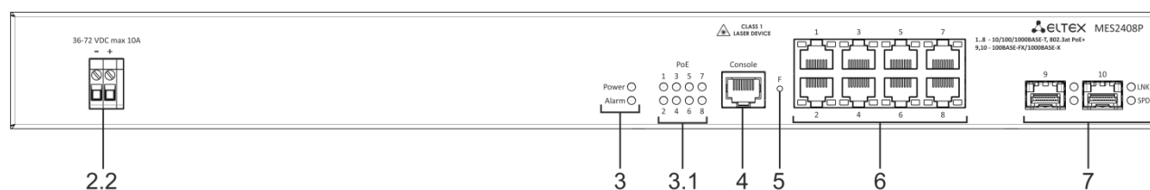
Рисунок 10 – Передняя панель MES2408P DC
