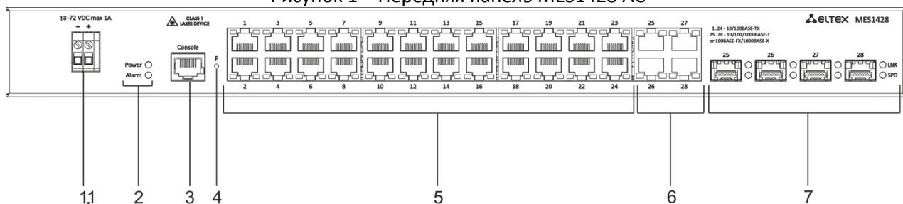
Рисунок 2 – Передняя панель MES1428 DC
