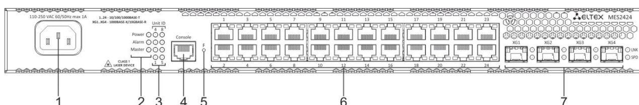
Рисунок 17 – Передняя панель MES2424 AC
