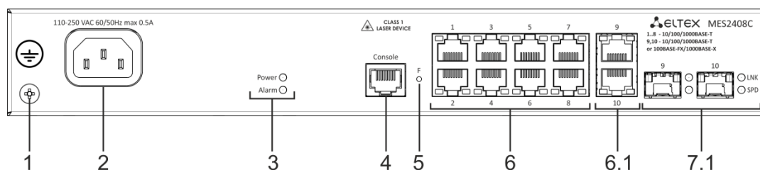
Рисунок 6 – Передняя панель MES2408C
