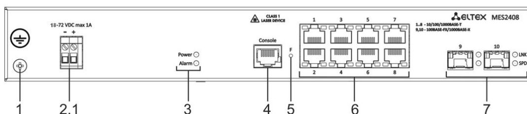
Рисунок 4 – Передняя панель MES2408 DC
