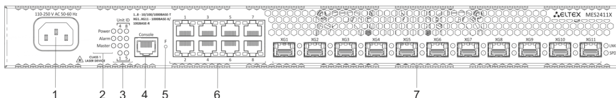
Рисунок 25 – Передняя панель MES2411X
