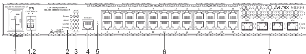
Рисунок 19 – Передняя панель MES2424B
