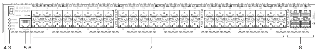
Рисунок 31 – Передняя панель MES3400-48F
