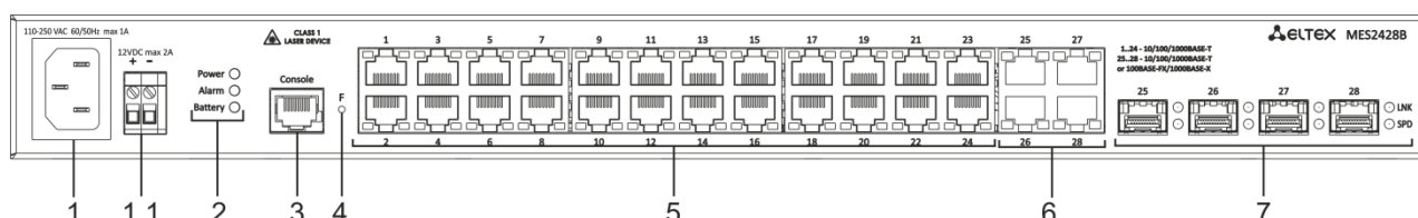
Рисунок 14 – Передняя панель MES2428B
