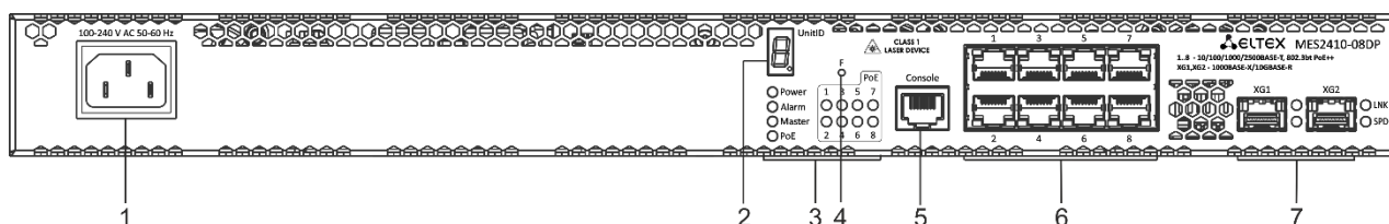
Рисунок 32 – Передняя панель MES2410-08DP
