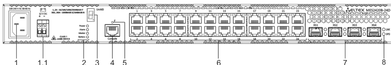
Рисунок 34 – Передняя панель MES2420B-24D
