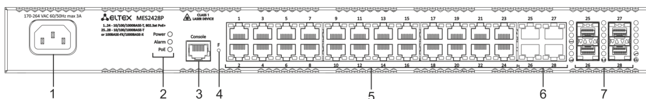
Рисунок 15 – Передняя панель MES2428P AC
