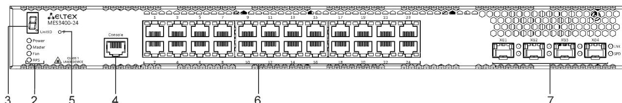
Рисунок 26 – Передняя панель MES3400-24
