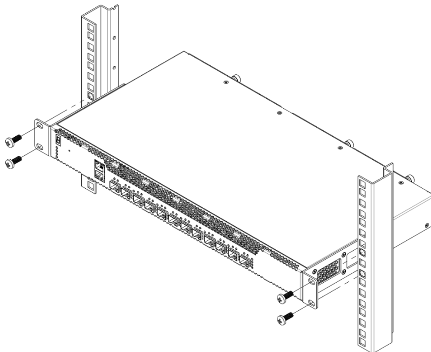
Рисунок 58 – Установка устройства в стойку
