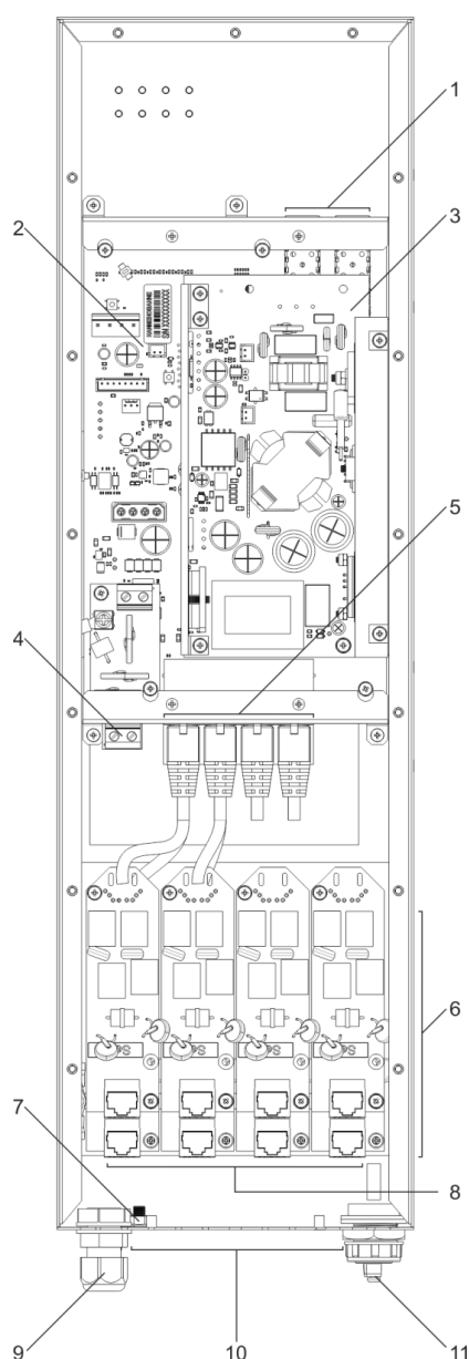
Рисунок 52 – Основные компоненты и разъемы MES3708P
