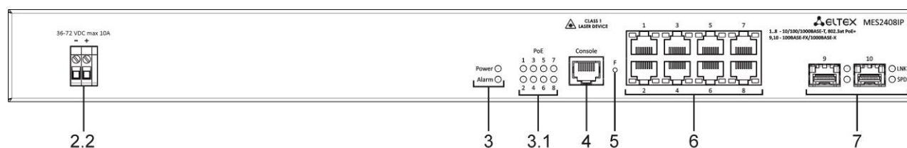
Рисунок 8 – Передняя панель MES2408IP DC1
