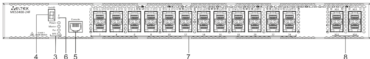
Рисунок 30 – Передняя панель MES3400-24F
