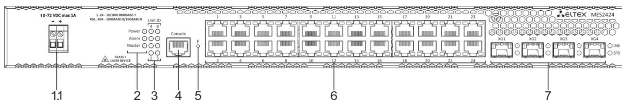
Рисунок 18 – Передняя панель MES2424 DC
