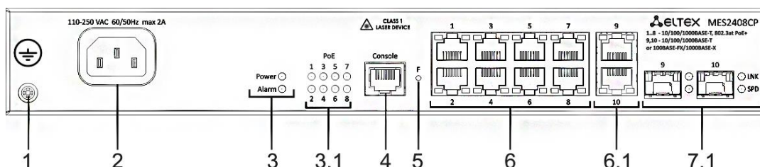
Рисунок 7 – Передняя панель MES2408CP
