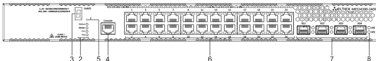
Рисунок 35 – Передняя панель MES2420D-24DP
