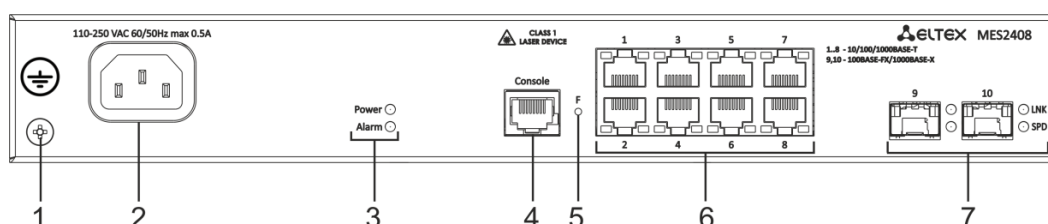
Рисунок 3 – Передняя панель MES2408 AC
