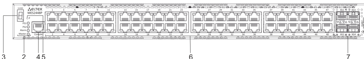
Рисунок 23 – Передняя панель MES2448P
