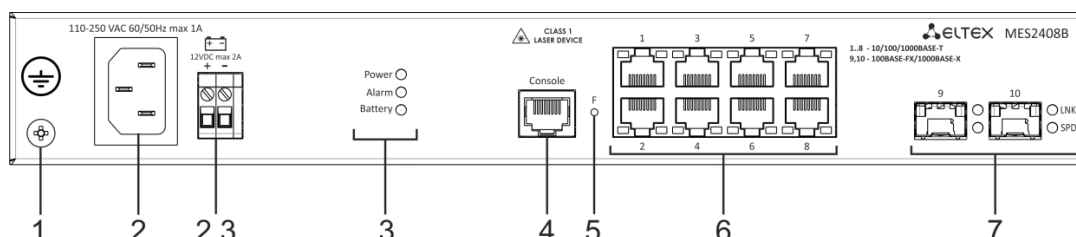
Рисунок 5 – Передняя панель MES2408B
