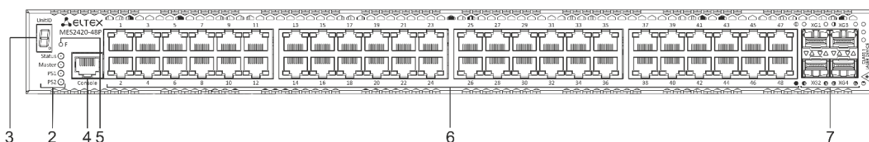
Рисунок 24 – Передняя панель MES2420-48P
