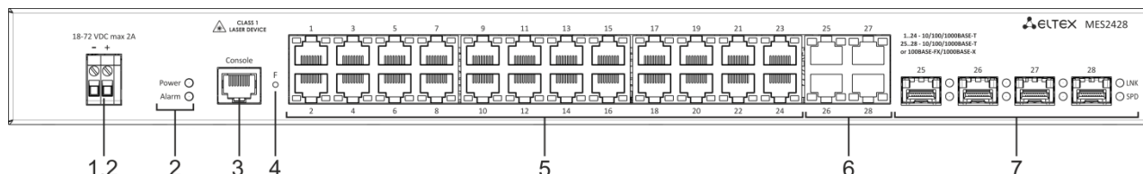
Рисунок 13 – Передняя панель MES2428 DC
