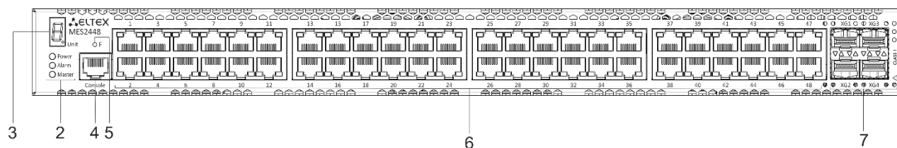
Рисунок 21 – Передняя панель MES2448 DC
