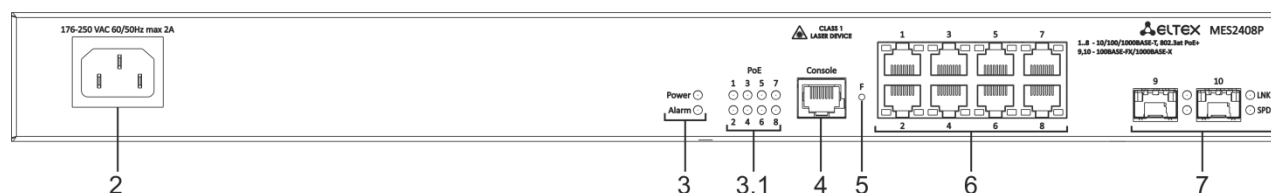
Рисунок 9 – Передняя панель MES2408P AC
