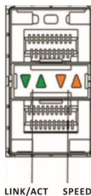
Рисунок 54 – Внешний вид сдвоенного разъема SFP/SFP+
