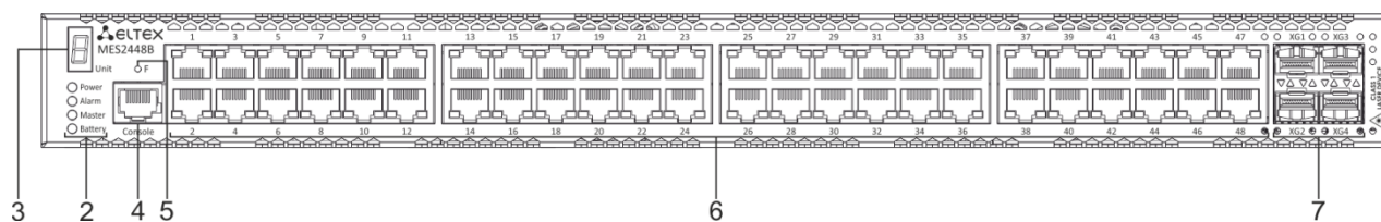
Рисунок 22 – Передняя панель MES2448B
