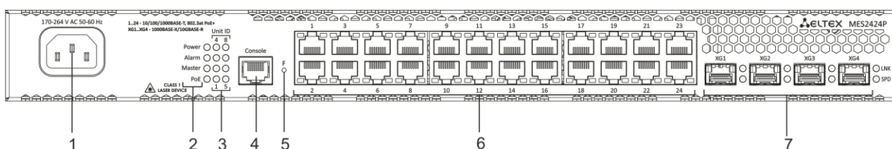
Рисунок 20 – Передняя панель MES2424P
