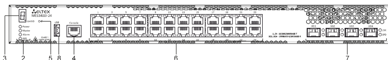
Рисунок 27 – Передняя панель MES3400I-24
