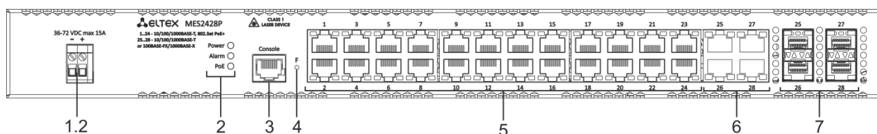
Рисунок 16 – Передняя панель MES2428P DC
