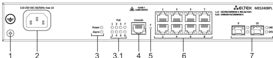
Рисунок 11 – Передняя панель MES2408PL
