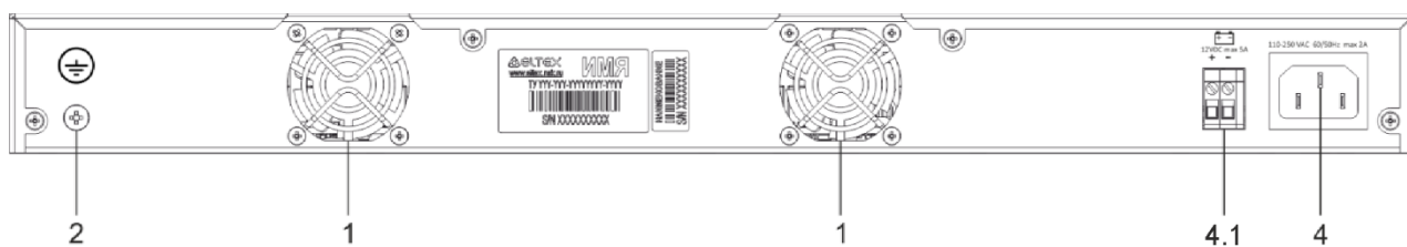
Рисунок 41 – Задняя панель MES2448B
