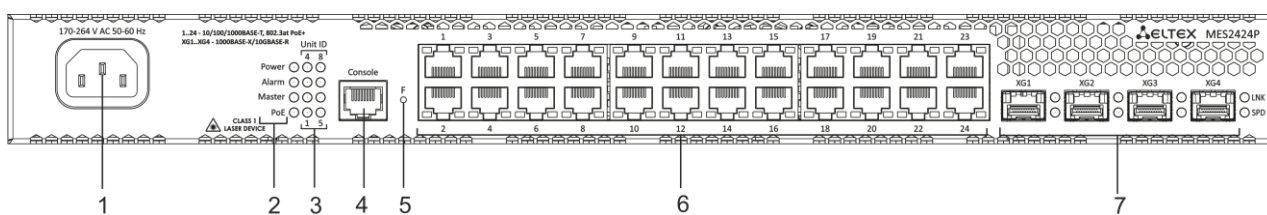
Рисунок 20 – Передняя панель MES2424P
