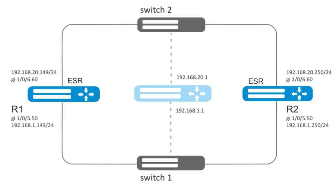
Рисунок 69 – Схема сети
