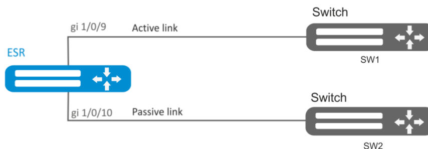
Рисунок 58 – Схема сети
