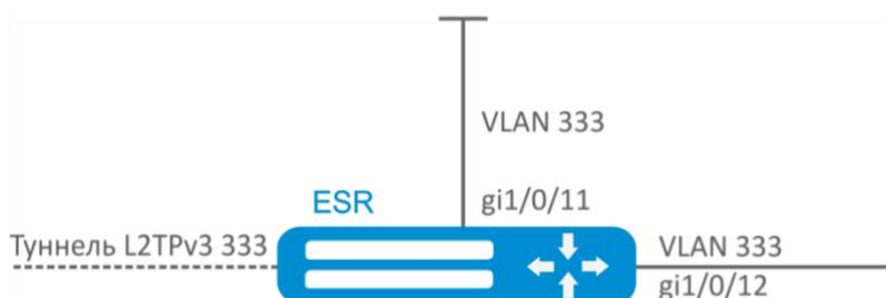
Рисунок 38 – Схема сети
