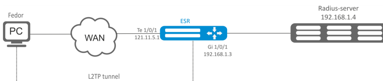
Рисунок 53 – Схема сети
