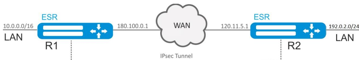
Рисунок 51 – Схема сети
