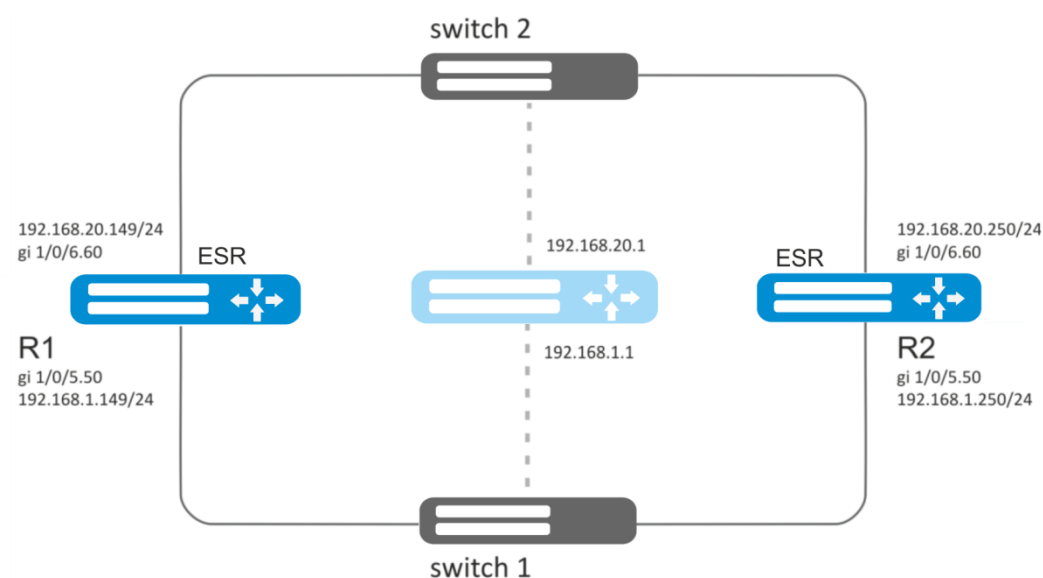
Рисунок 66 – Схема сети
