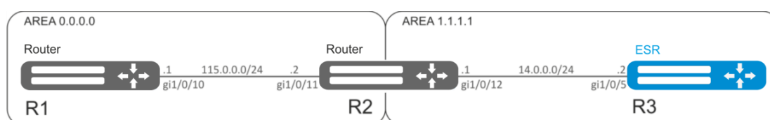
Рисунок 42 – Схема сети
