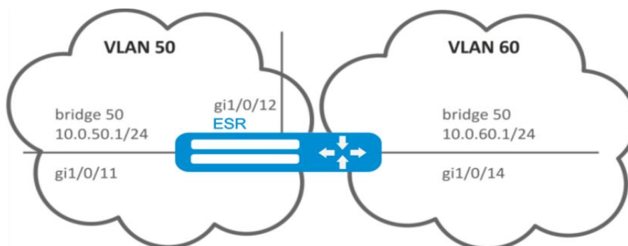
Рисунок 39 – Схема сети
