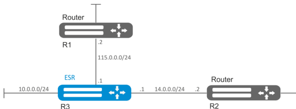
Рисунок 40 – Схема сети
