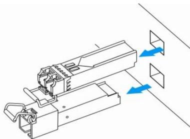
Рисунок 20 – Извлечение SFP-трансиверов
