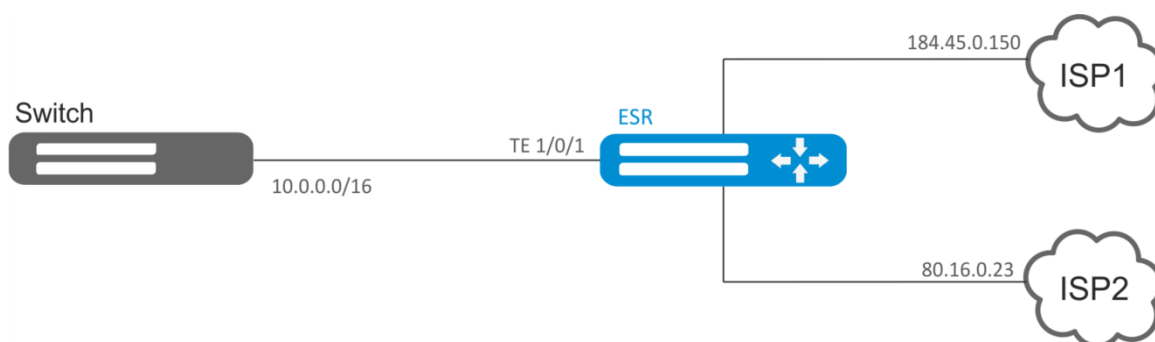
Рисунок 47 – Схема сети
