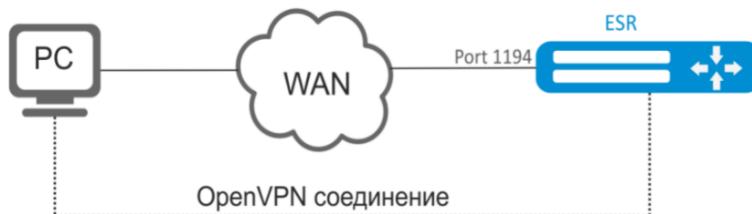
Рисунок 54 – Схема сети
