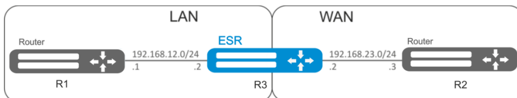
Рисунок 33 – Схема сети
