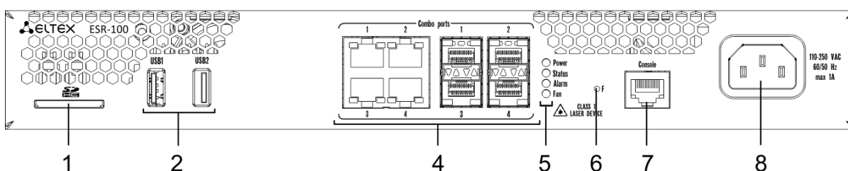
Рисунок 6 – Передняя панель ESR-100
