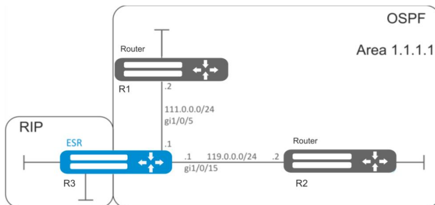
Рисунок 41 – Схема сети
