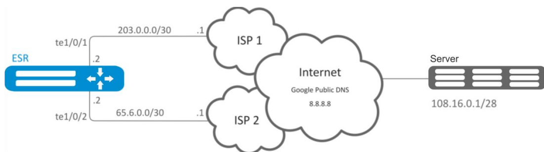
Рисунок 69 – Схема сети
