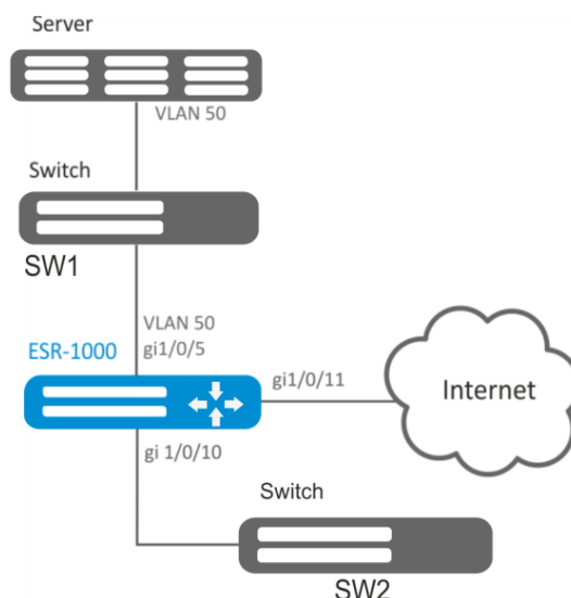
Рисунок 61 – Схема сети
