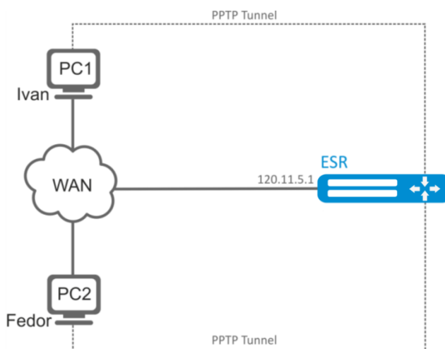
Рисунок 52 – Схема сети
