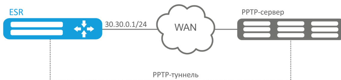
Рисунок 56 – Схема сети
