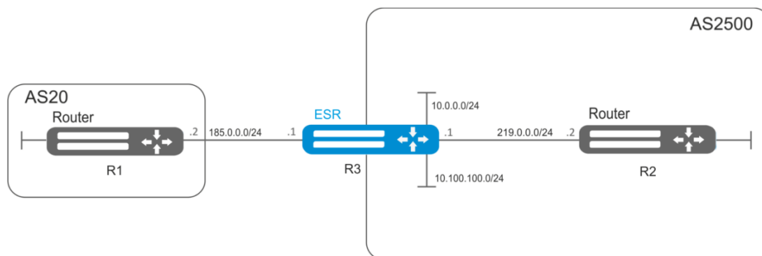
Рисунок 46 – Схема сети
