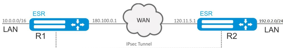
Рисунок 50 – Схема сети
