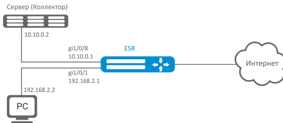
Рисунок 62 – Схема сети
