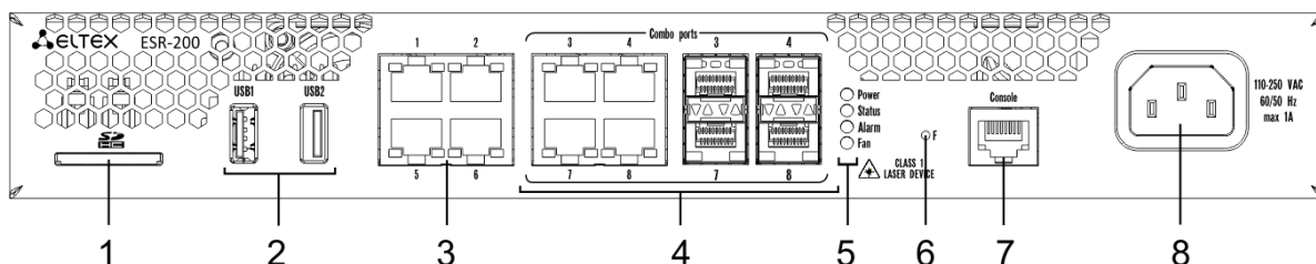
Рисунок 5 – Передняя панель ESR-200
