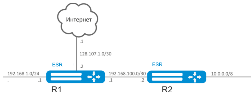
Рисунок 34 – Схема сети
