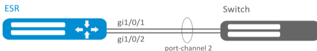
Рисунок 64 – Схема сети
