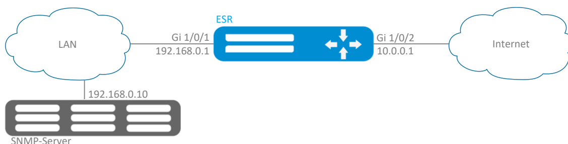
Рисунок 32 – Схема сети
