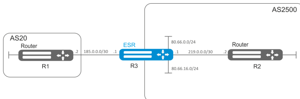
Рисунок 44 – Схема сети
