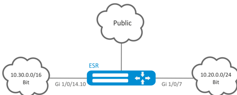
Рисунок 68 – Схема сети
