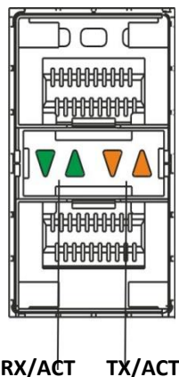
Рисунок 11 – Расположение индикаторов оптических интерфейсов
