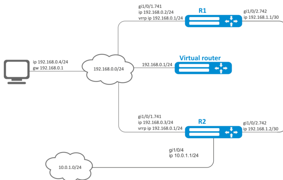
Рисунок 67 – Схема сети
