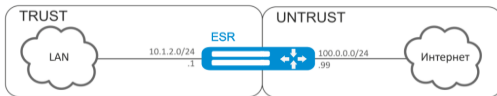
Рисунок 27 – Схема сети
