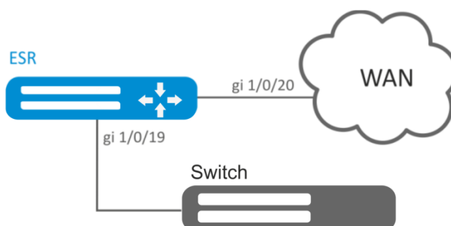
Рисунок 60 – Схема сети
