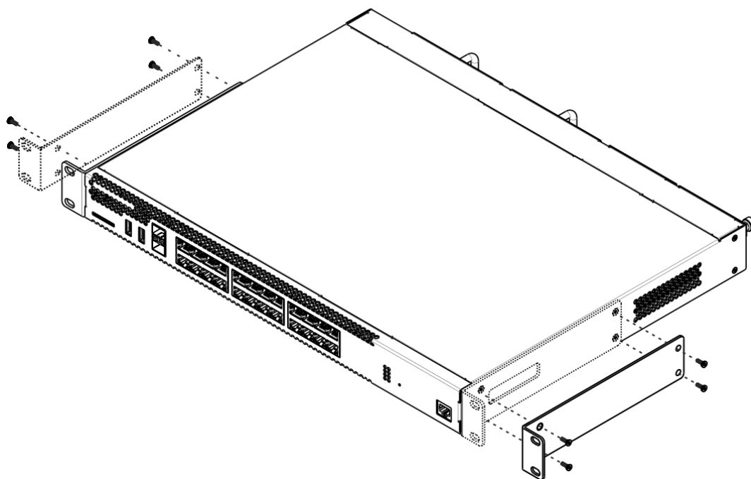
Рисунок 13 – Крепление кронштейнов
