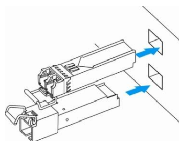
Рисунок 17 – Установка SFP-трансиверов
