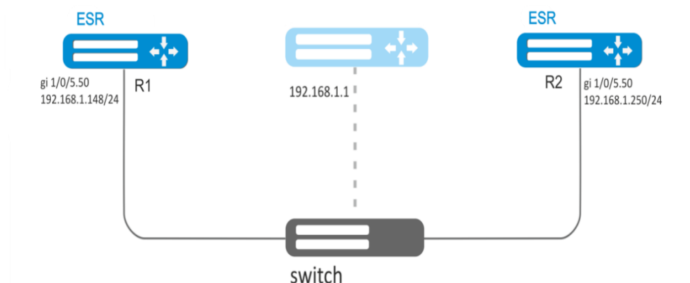
Рисунок 65 – Схема сети
