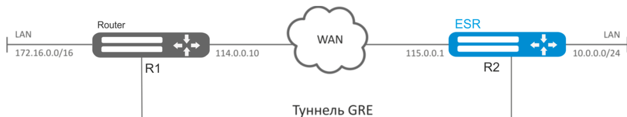
Рисунок 48 – Схема сети
