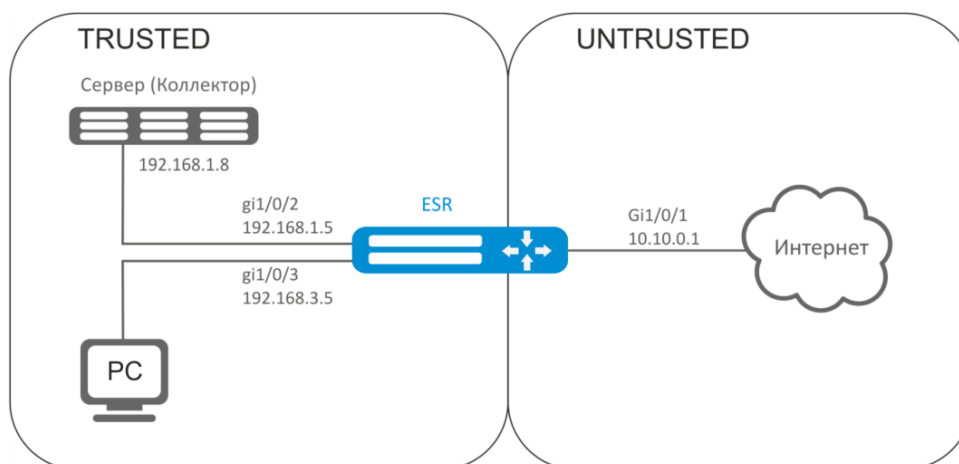
Рисунок 63 – Схема сети
