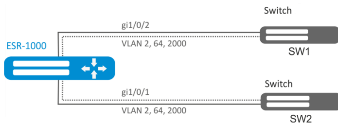
Рисунок 22 – Схема сети
