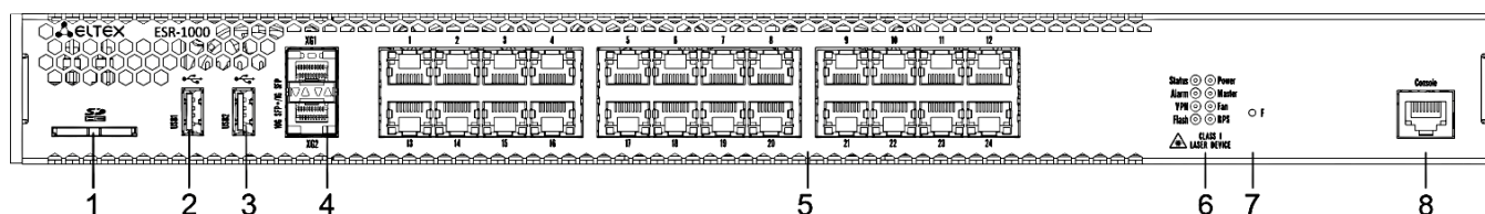
Рисунок 1 – Передняя панель устройства ESR-1000
