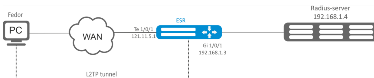
Рисунок 53 – Схема сети
