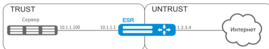
Рисунок 26 – Схема сети
