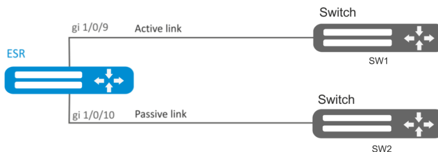
Рисунок 58 – Схема сети
