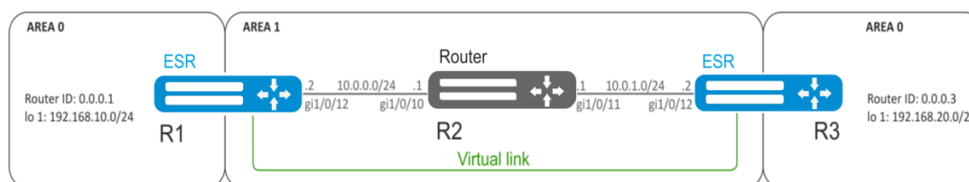
Рисунок 43 – Схема сети
