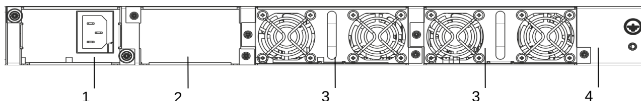
Рисунок 2 – Задняя панель ESR-1000
