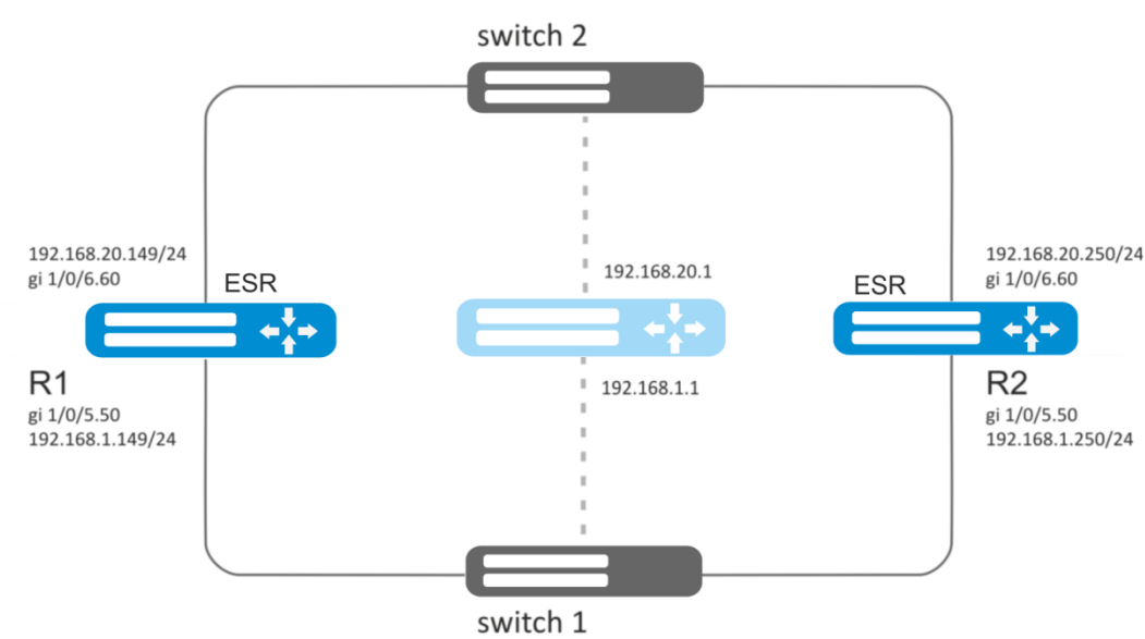
Рисунок 10.32 – Схема сети
