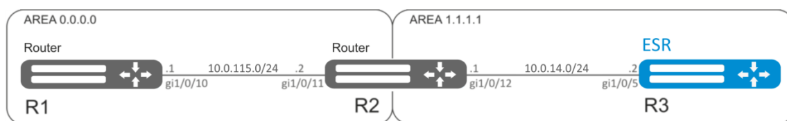
Рисунок 10.16 – Схема сети
